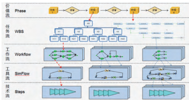
图5 五层精益流程模型
