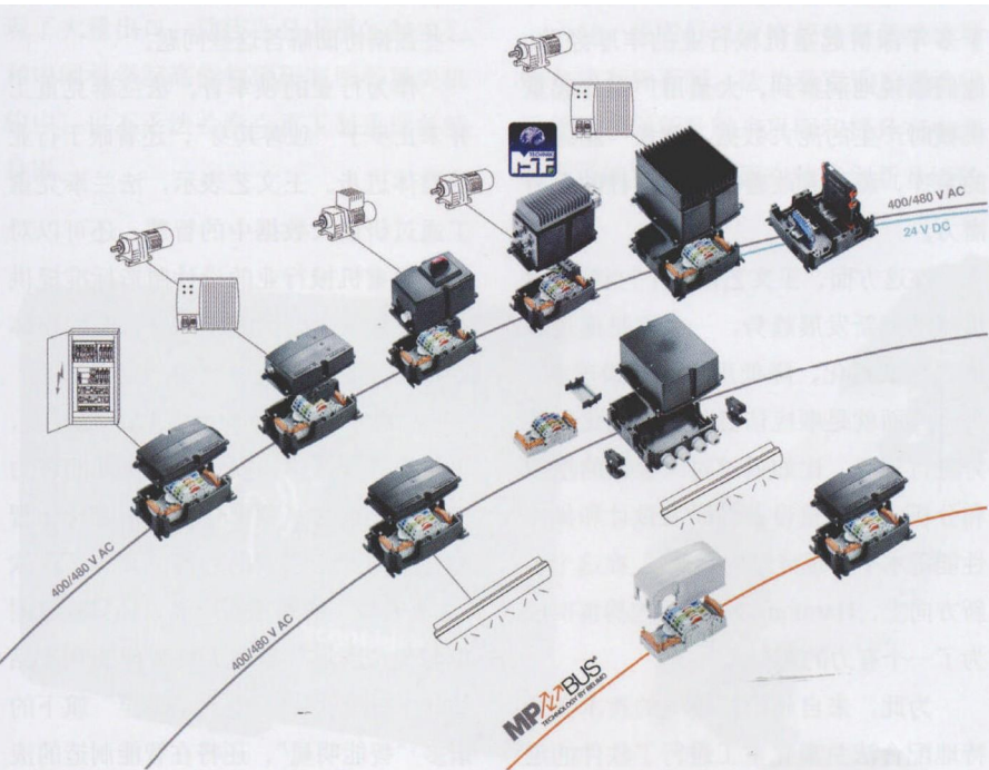
图 魏德米勒 Fieldpower® 在智能化输送线馈电分配的应用 719
