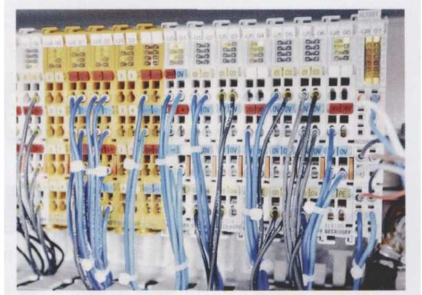
图3 通过 Twinsafe 端子模块 (中) 和伺服电机 Ethercat 端子模块 EL7201 (右) 可以将安全和驱动技术无缝并紧凑地集成到控制系统中
