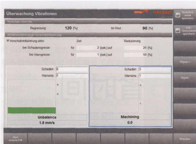
图1 通过采用适应性强的“闲聊控制”进给调节功能，可以提高生产流程的安全性并降低刀具的磨损程度
