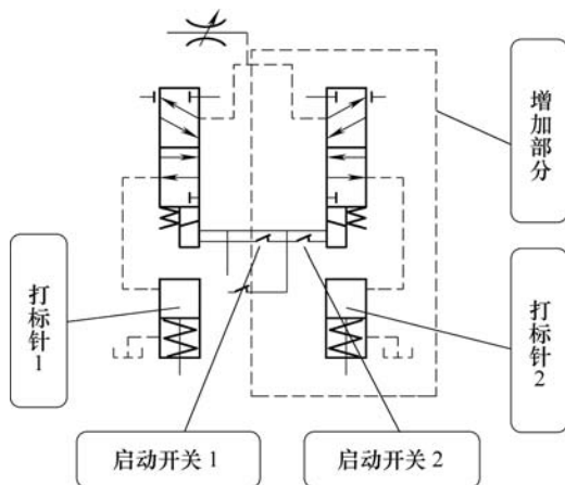
图2 电气控制原理图
