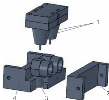
图1 机械结构示意图
