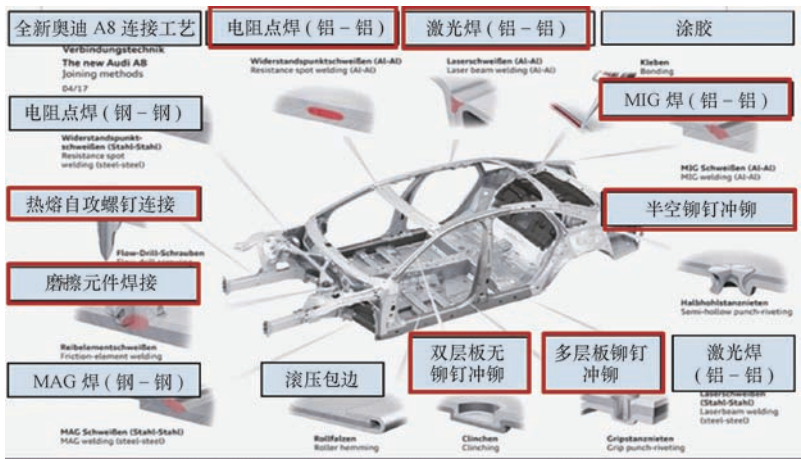
图2 2A8车身的连接工艺
