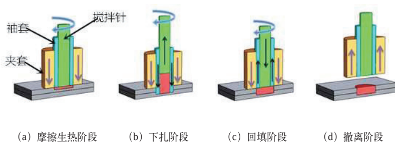
图7 搅拌摩擦焊原理
