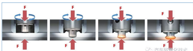
图5 摩擦元件焊接工作原理
