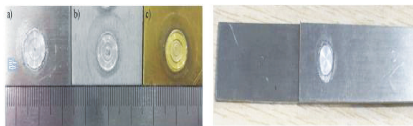
图6 搅拌摩擦点焊
