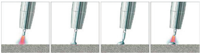
图3 冷金属过渡焊
