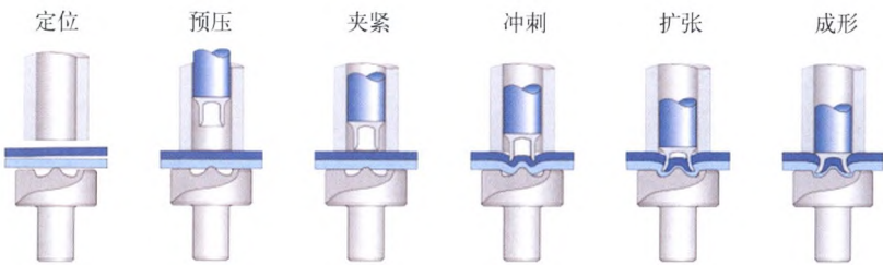
图2 SPR工艺过程
