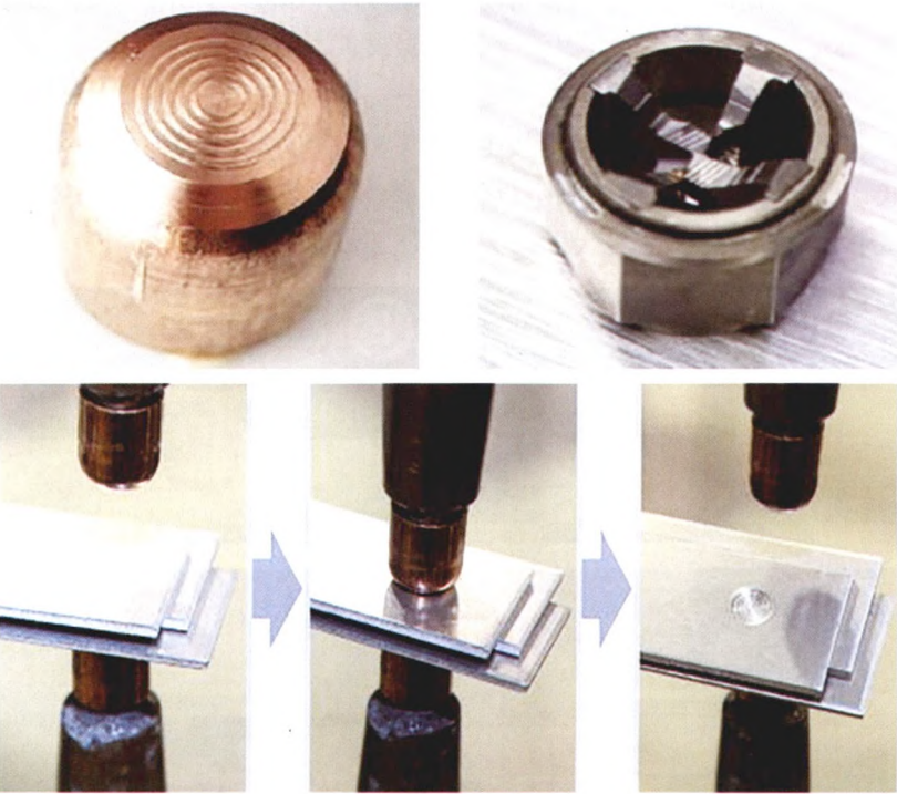
图7 螺旋状电极铝合金点焊
