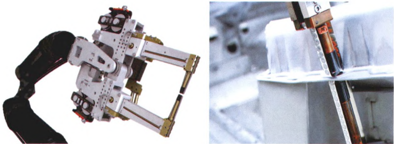
图8 电极带式铝点焊
