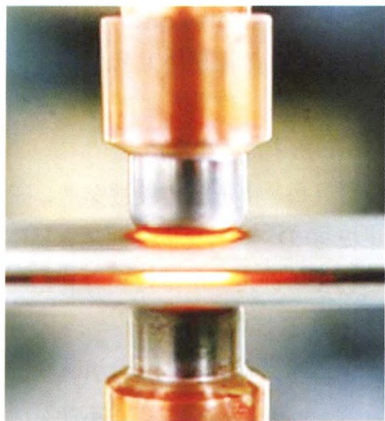
图6 常规铝合金点焊
