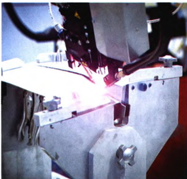
图11 激光填丝焊
