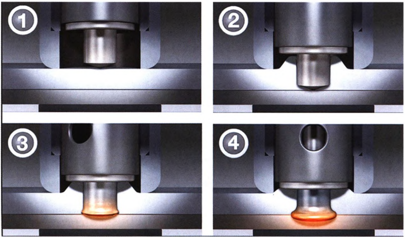
图4 EJOWELD工艺原理
