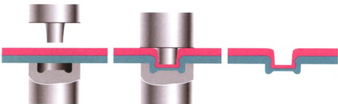
图3 Clinchen工艺原理
