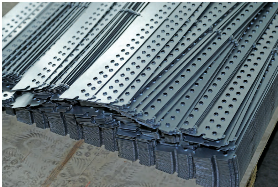
图2 经过纵横各一次的矫平，在短短几分钟内，昶浩泰的不锈钢钣金件的平整度就从原来的2mm顺利降至要求的0.01mm
