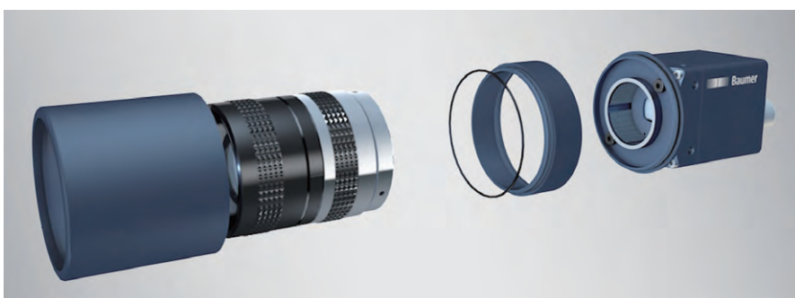
图 1 相机配备已获专利的模块化镜头保护套管系统（可选 M47 或 M62 螺纹），支持各种规格的套管扩展圈，能够为不同长度、不同直径的镜头提供快速灵活的保护，确保防护等级达到 IP54、IP65 和 IP67
