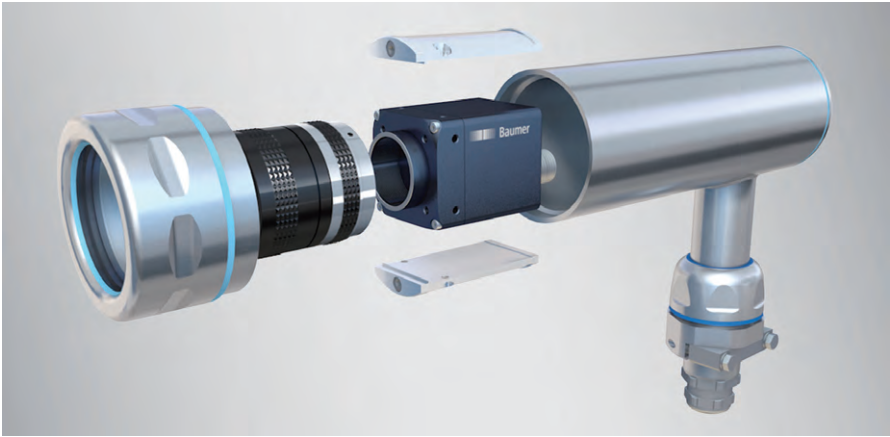
图 3 IP69K 防护外壳采用卫生型不锈钢设计，残留介质没有任何可乘之机粘附在相机表面
