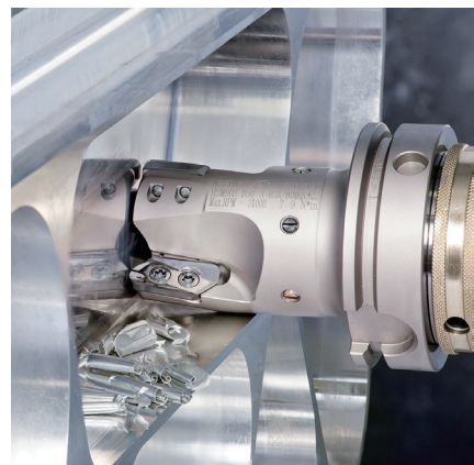
图 4 这一概念保证在转速高达 31 000 r/min 时也能执行可靠的铣削加工
