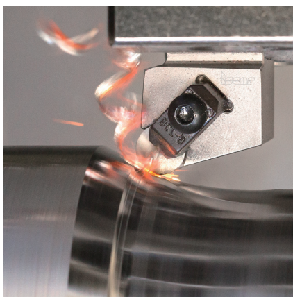
图 1 伊斯卡开发出新的“TE”切削刀口形状，以提高在粗加工和断续切削这类重载条件下的刀具寿命
