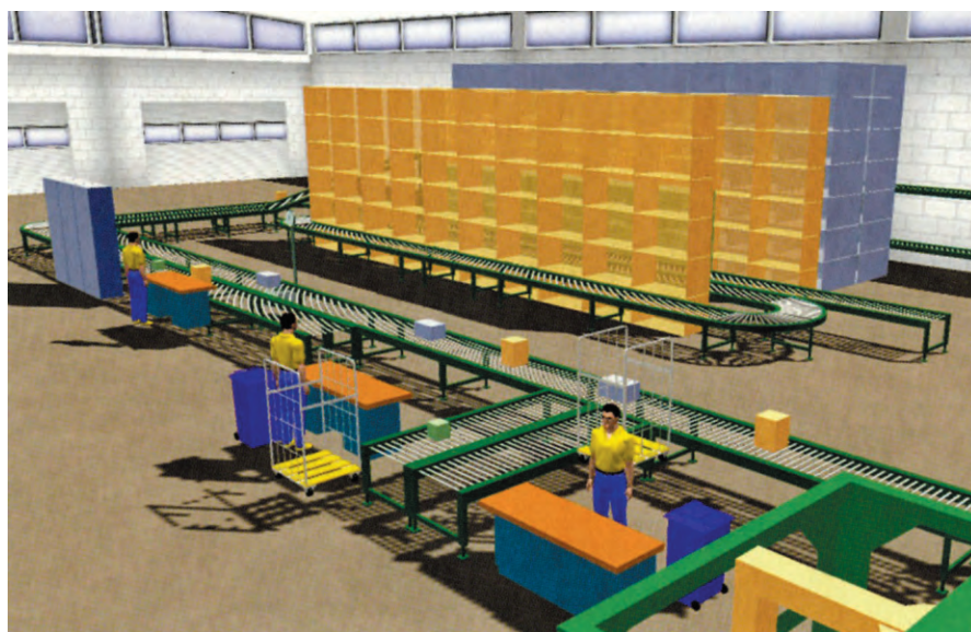
图 2 生产区材料流的优化
