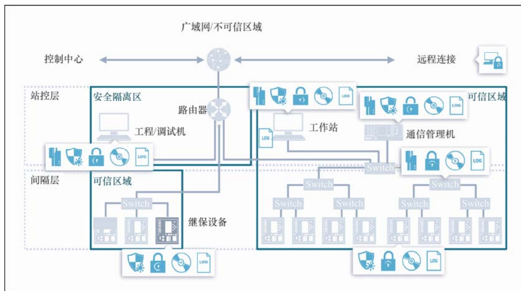
图2 电力系统整体安全框架
