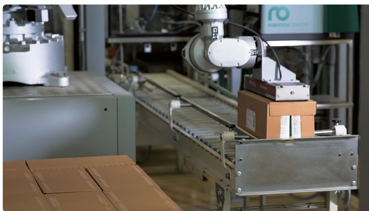
利用胶条对二次包装进行码垛
