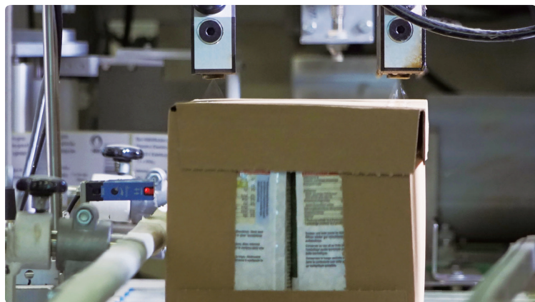
两个 AX Diamond 型喷枪在喷涂胶粘剂
