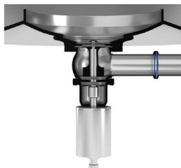
图 1 搅拌机卡箍具密封件的安装情况
