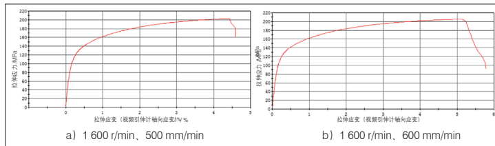
图6 拉伸应变曲线
