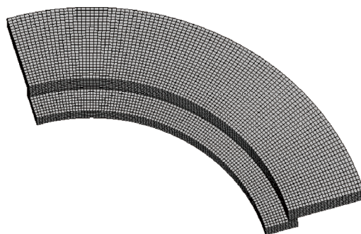
图3 网格划分
