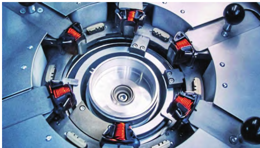
图 1 在生产单元中，SMC 的电动缸负责部件的定位和过程受到监控的推力操作
