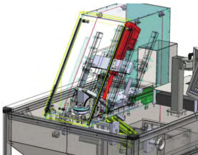
图 3 Riedmayer Engineering & Maschinenbau 公司的两个装配和折弯站设计精巧，可实现涡轮增压器电驱动生产的自动化
