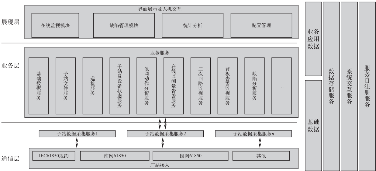
图2 系统平台架构
