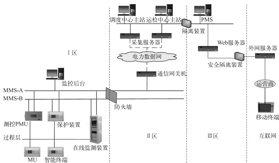
图1 网络架构
