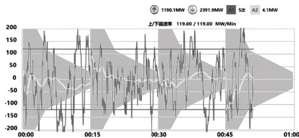
图 12 ACE 实时考核监视告警
