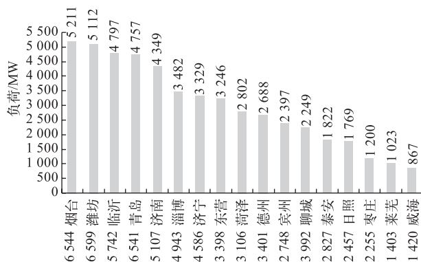
图2 地区用电负荷(柱图)
