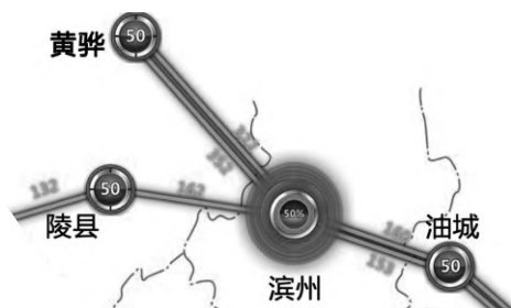
图10 暂态失稳告警信息展示
