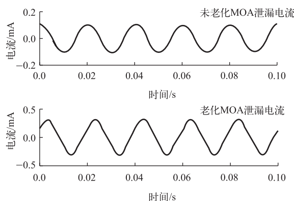
图2 MOA老化前后的泄漏电流仿真波形（无干扰）
