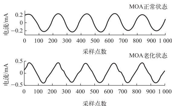
图7 MOA泄漏电流实测信号去噪结果
