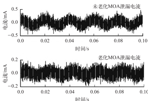
图3 MOA老化前后的泄漏电流仿真波形（有干扰）
