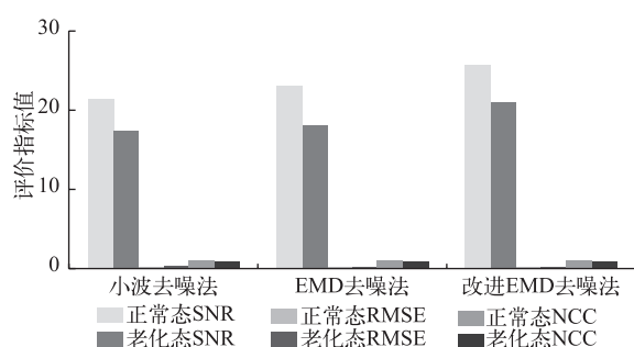
图8 不同方法下 MOA 泄漏电流去噪结果
