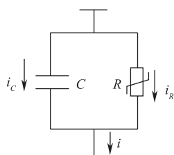
图1 MOA等效模型图
