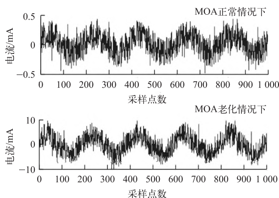
图6 MOA泄漏电流实测信号结果
