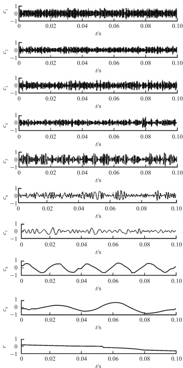
图4 MOA 老化后的泄漏电流 IMF 分量
