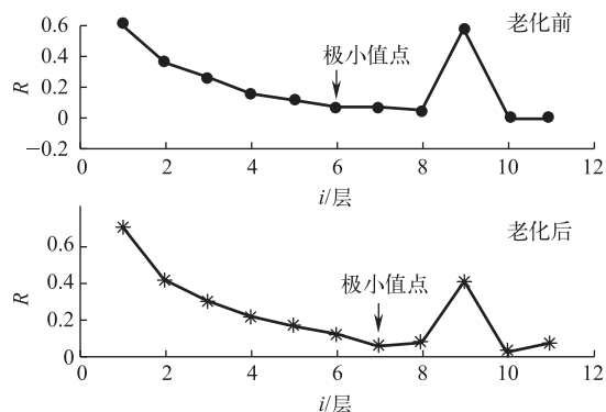
图5 MOA老化前后的泄漏电流模态分界点
