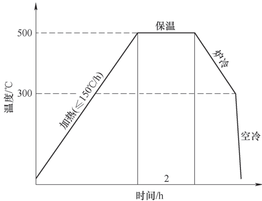
图2 P91钢退火工艺曲线
