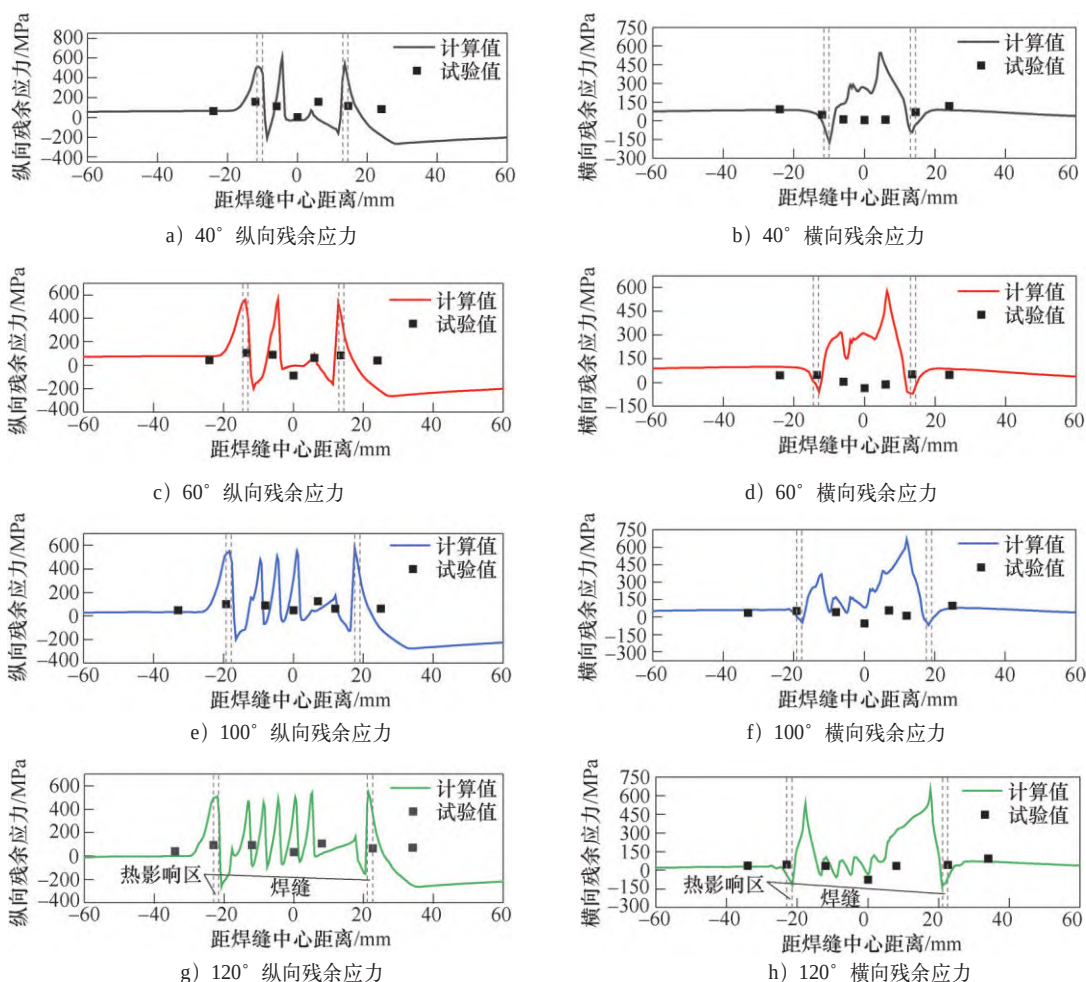
图8 各坡口角度上表面残余应力计算值与试验值对比
