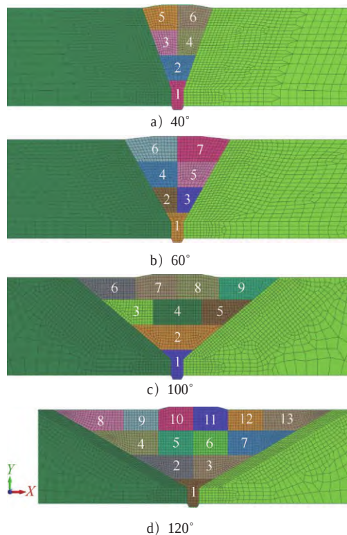
图4 有限元网格模型
