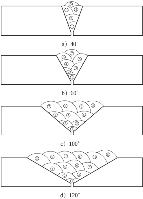
图3 不同坡口角度的焊道布置
