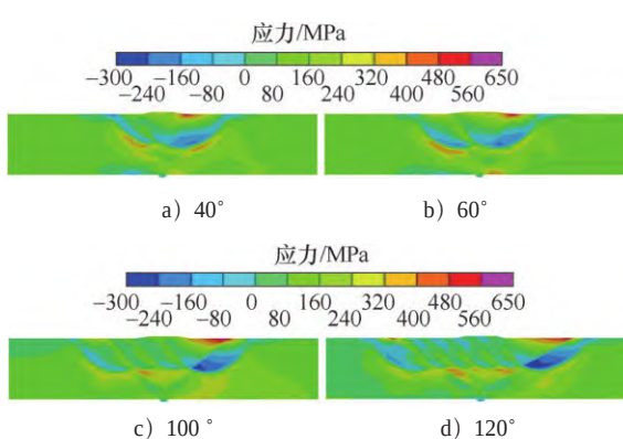
图10 不同坡口角度横向残余应力分布云图
