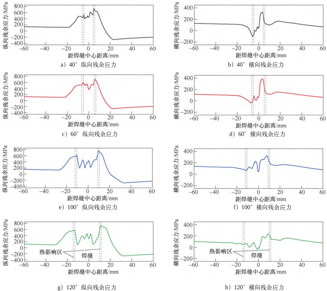
图11 接头下表面纵向和横向残余应力分布曲线
