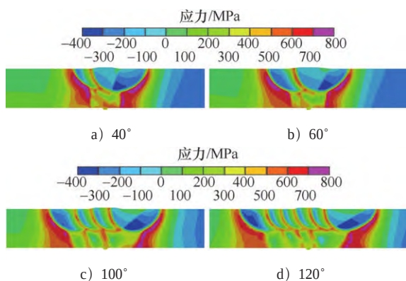
图9 不同坡口角度上表面纵向残余应力分布云图
