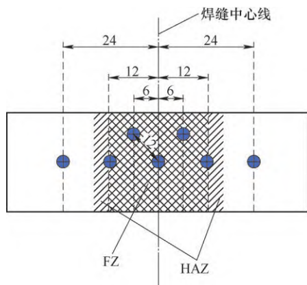
a) 上表面焊接接头应力测点位置
