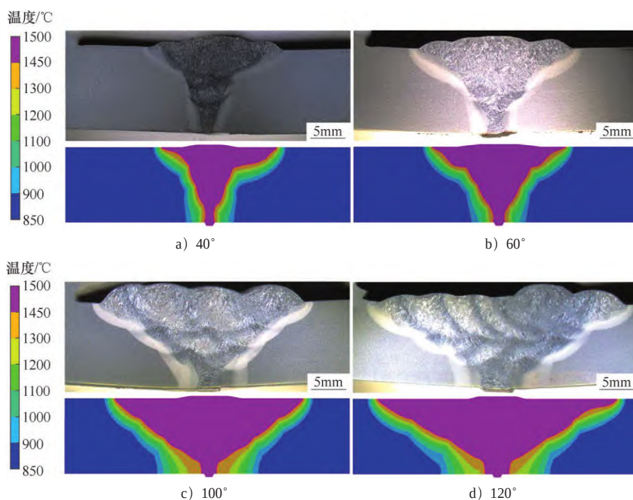
图5 校核完成后的模拟结果与实际焊缝几何形状对比
