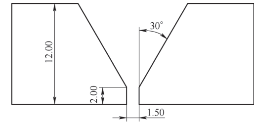
图1 V形坡口
