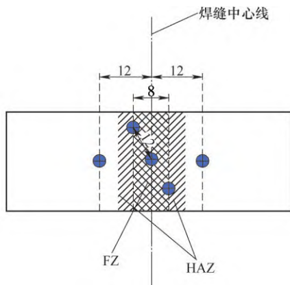
b) 焊接接头下表面应力测点位置
