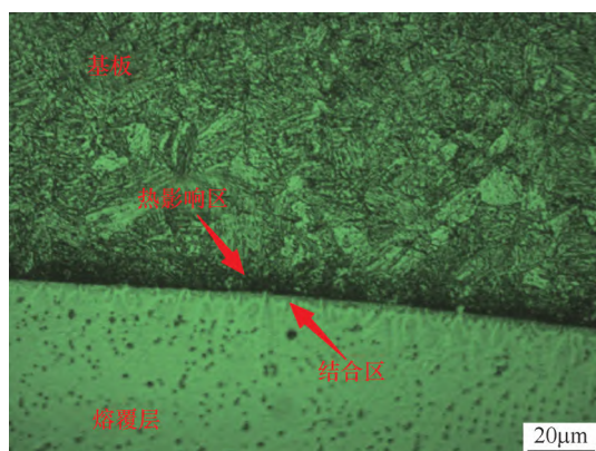
a) 结合区域 (500×)
