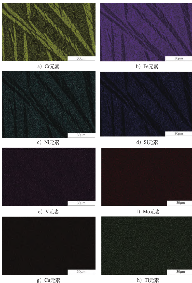
图5 熔覆层面扫描结果
