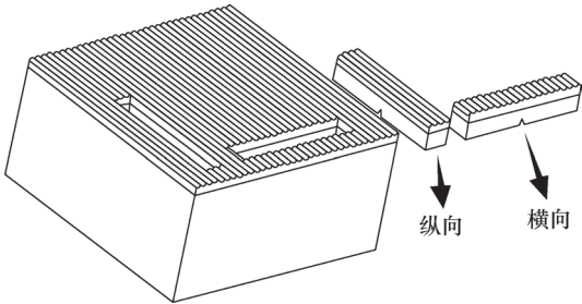
图2 冲击试样取样位置及缺口位置
