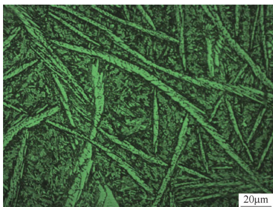
b) 熔覆层 (500×)
