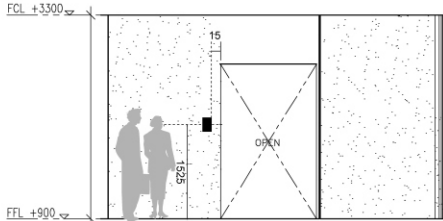
ELEVATION 立面 Scale 比例 1:50 Elevation for reference only. Not actual elevation.
