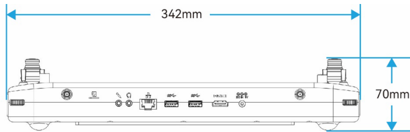
图 2 侧视图
