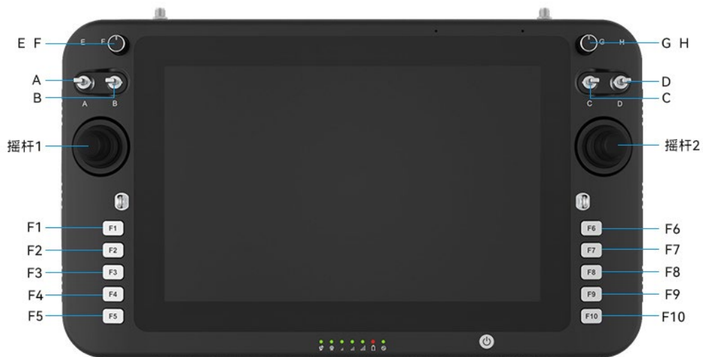
图 5 地面站扩展接口位置图
