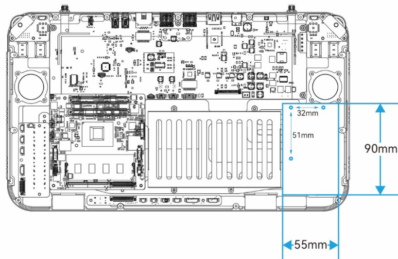
图 3 预留尺寸 90*55*18mm (最大) , 三个预留安装孔中心距:51*32mm
