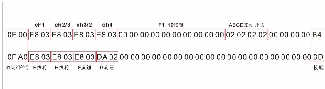
图 6 协议帧含义
