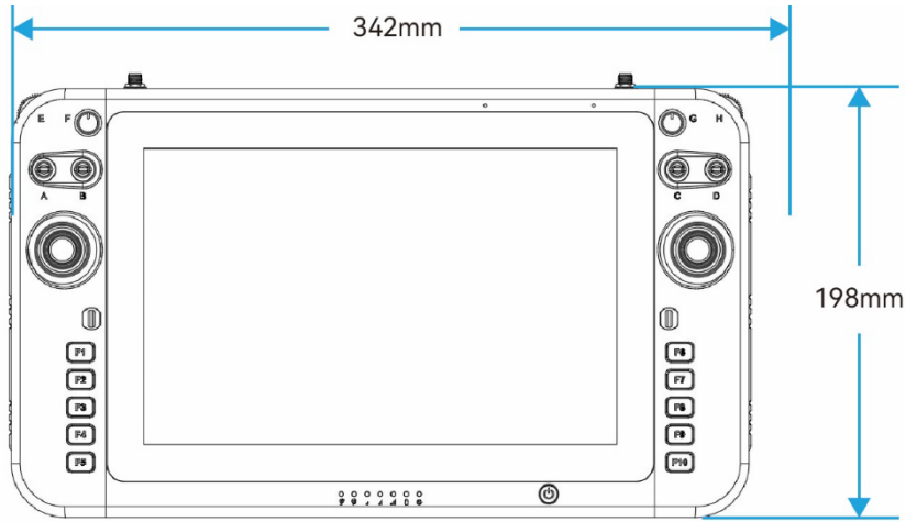
图 1 顶视图
