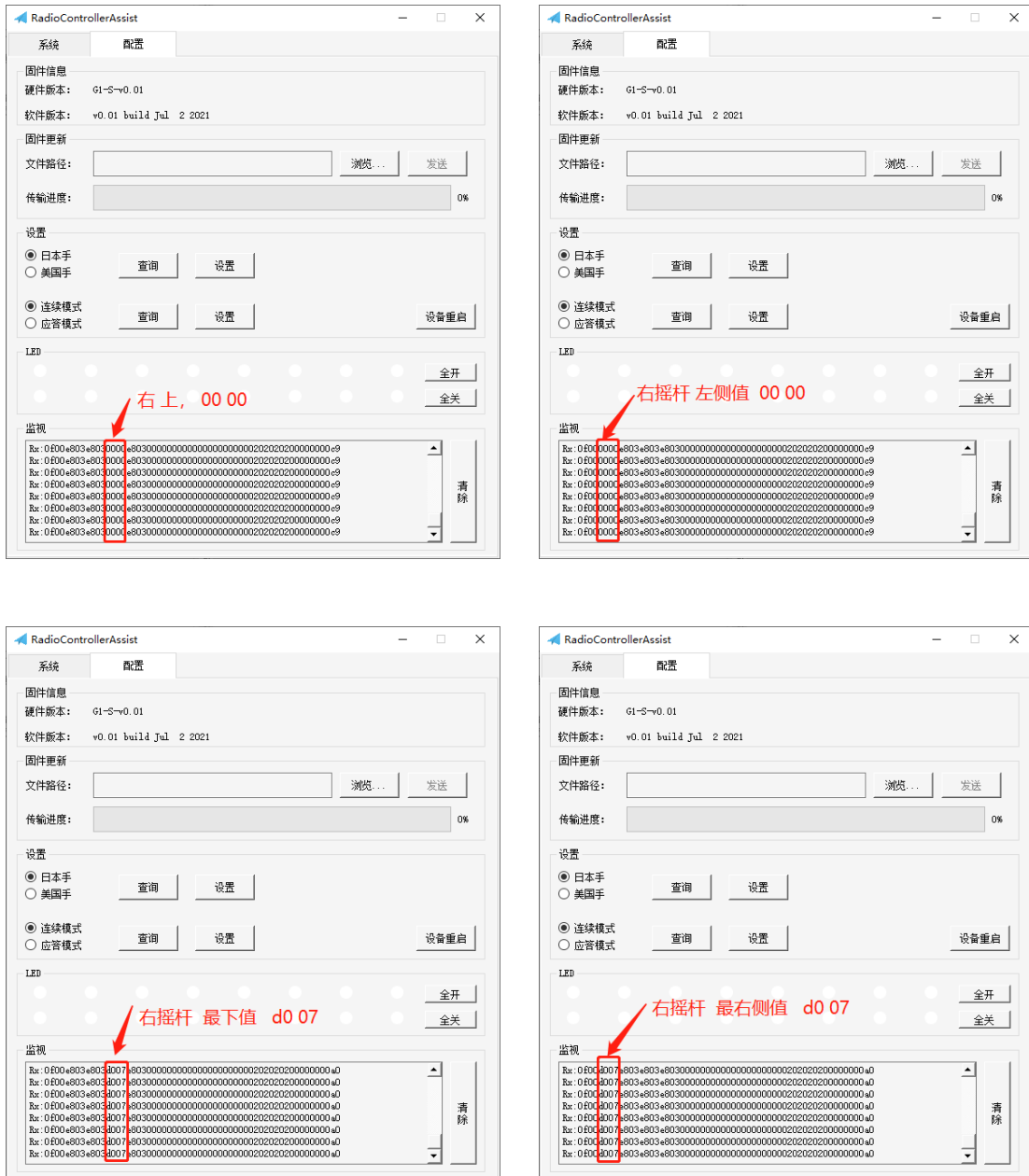
摇杆 2-右侧摇杆四个方向极限值与协议对应位置
