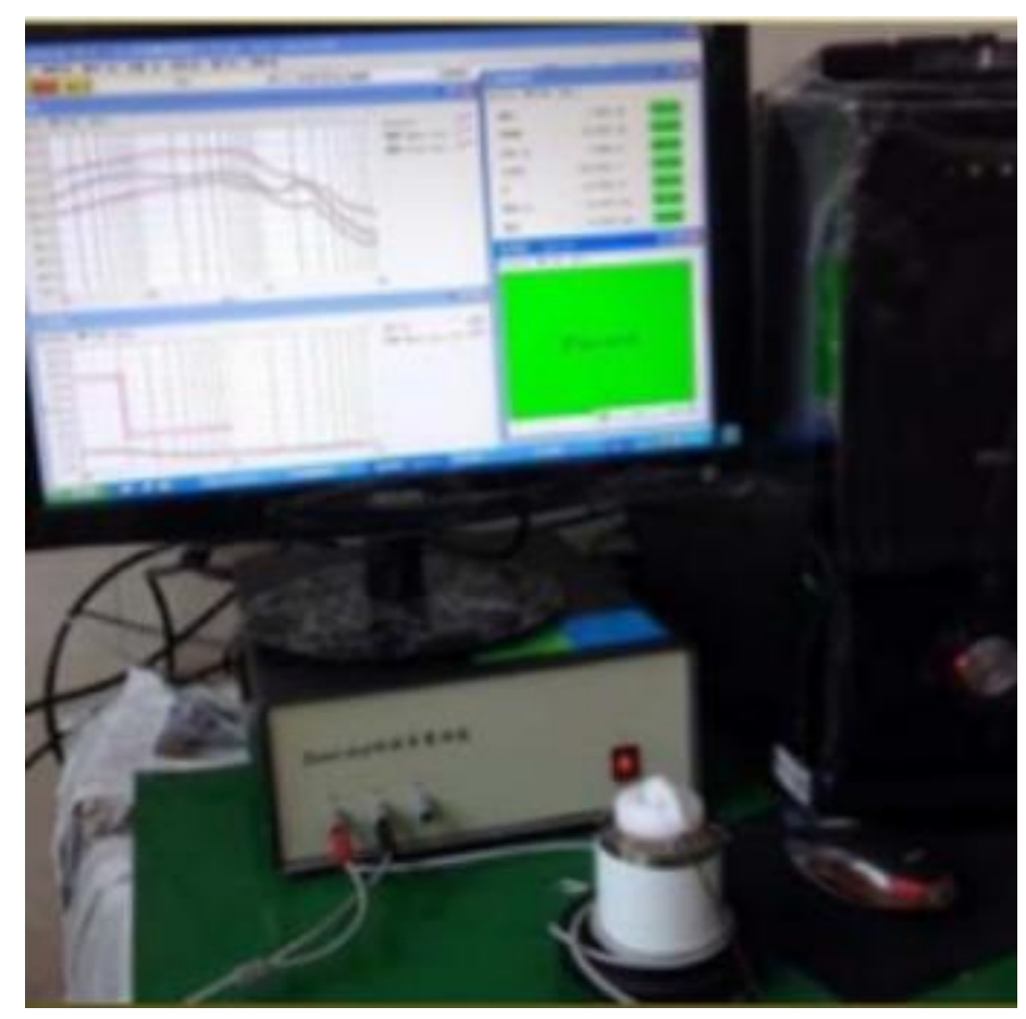
Soundcheck曲线测试仪
