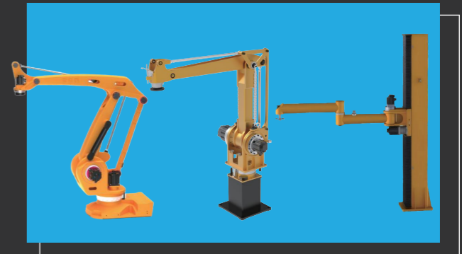
搬运、码垛多关节机器人
