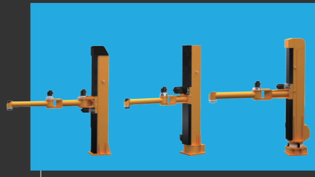
视觉拆垛破包投料专机
