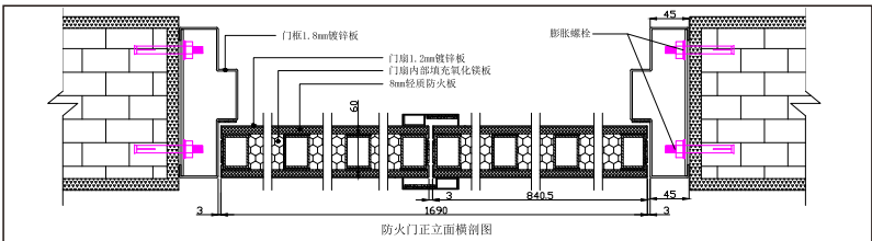
超大防火门结构图
