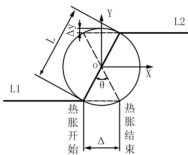
图2 Π型组合补偿器平面图
