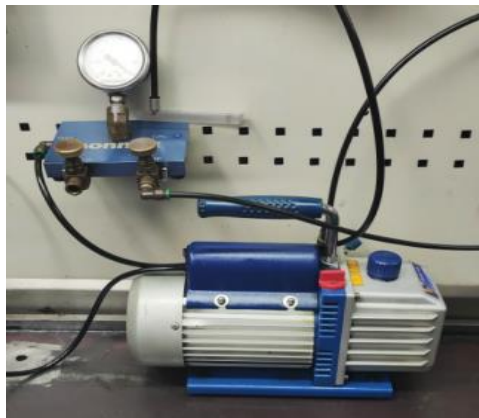
真空测漏仪
