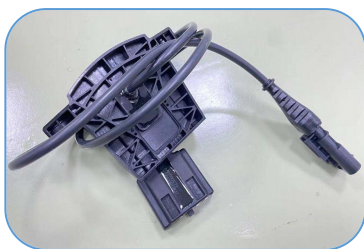
线性位移传感器壳体 用于离合器, PRD档位置检测等 Pin针、铜套、磁铁嵌件注塑
