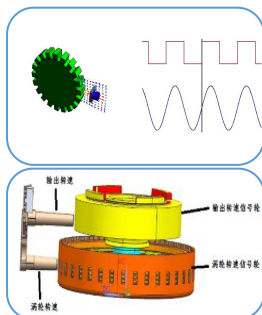
速度传感器骨架与包胶模 ABS轮速, 发动机齿轮, 变速箱齿轮等速度检测 Leadframe 嵌件注塑、芯片电阻焊后包胶注塑 Pin针铜套嵌件注塑
