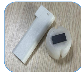
液位传感器壳体 检测冷却液, 雨刮水等液位 Pin针、磁铁嵌件注塑
