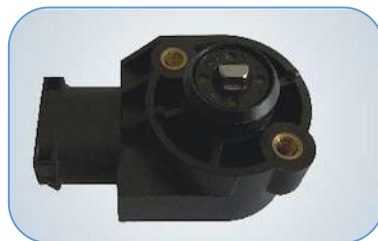
角度传感器壳体 刹车踏板, 油门踏板角度检测, 无人驾驶车轮方向检测等. 鱼眼Pin针、铜套、转动轴铜套嵌件注塑
