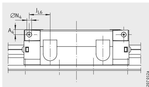
从侧面连接润滑接头
