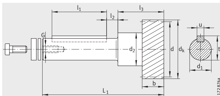
RITZ...-PF 键连接
