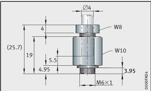
带活接头螺母接头, 螺母对边宽度 W_8 = 8 mm、 W_{10} = 10 mm
