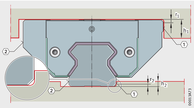
图 12 定位台阶高度和边角半径
