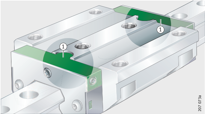
图 7 无上润滑孔的端盖
