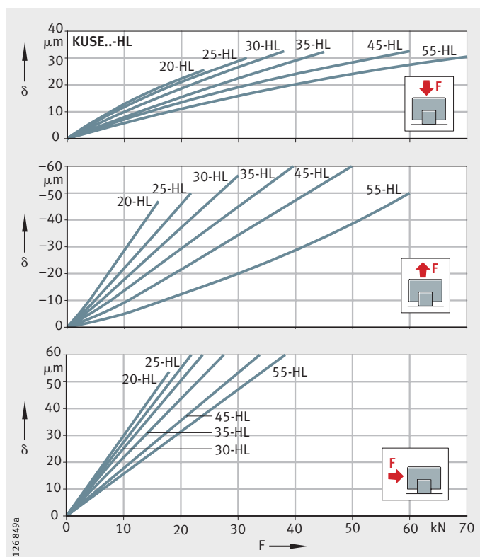
图 6 压、拉及侧向载荷下的弹性曲线
