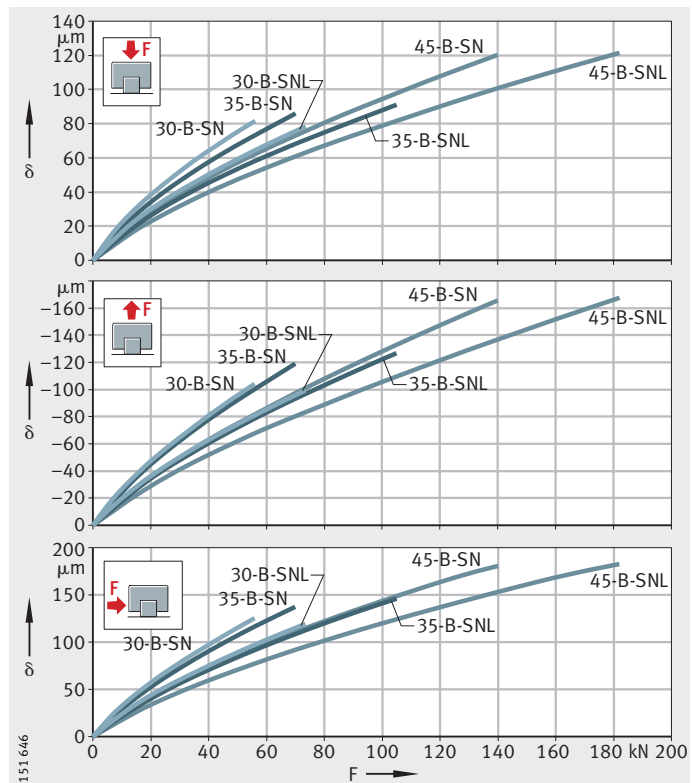
图 15 压力、拉力和侧向力作用下的 弹性曲线
