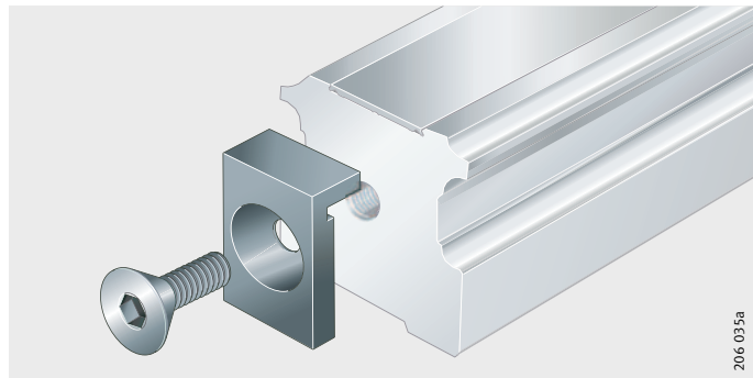
图 3 固定板
