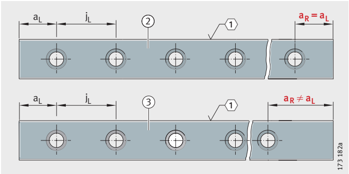
① 定位面 ② 对称螺栓孔形式 ③ 非对称螺栓孔形式 图 3 导轨螺栓孔形式 单列螺栓孔
