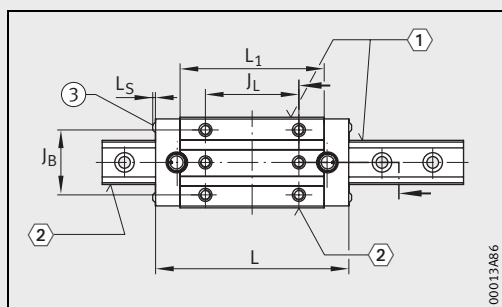
RUE...-E-KT-HL · 视图旋转 90° ①、②、③ 4)
