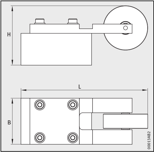
嵌入安装装置 ERVW
