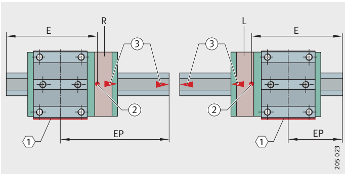
图 5 参考点的位置
