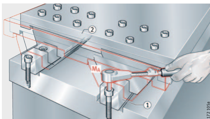
图 27 安装调整端
