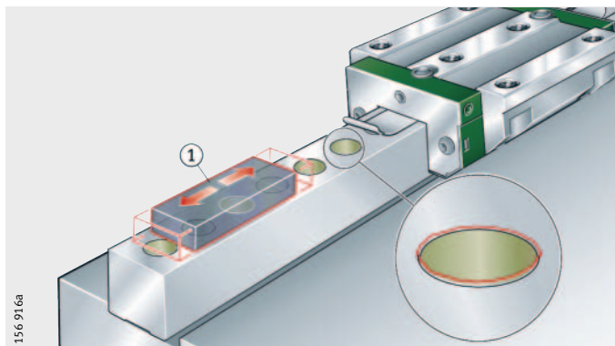
图 11 磨平填塞片
