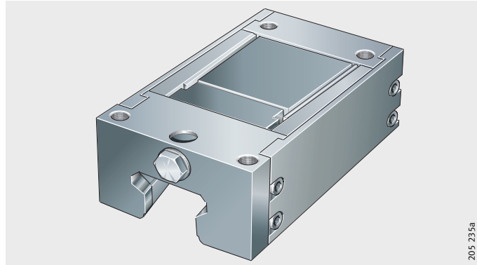
图 7 锁紧滑块
