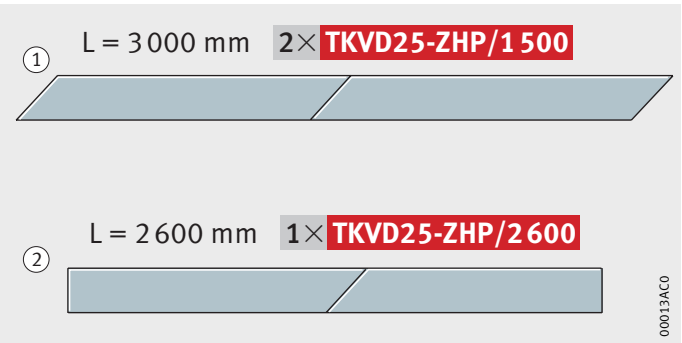
① 导轨端面为斜口 ② 导轨端面为直口 图 2 导轨的开始和结束端 为斜口或者直口
