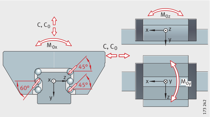
图 1 承载能力与接触角
