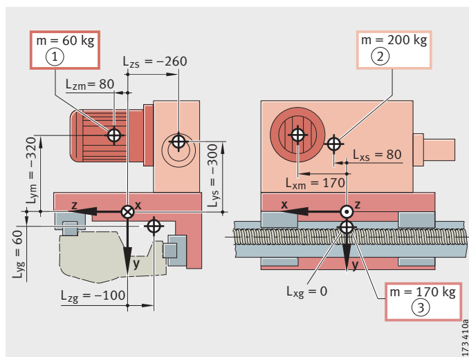
图 7 定义各组件重心位置
