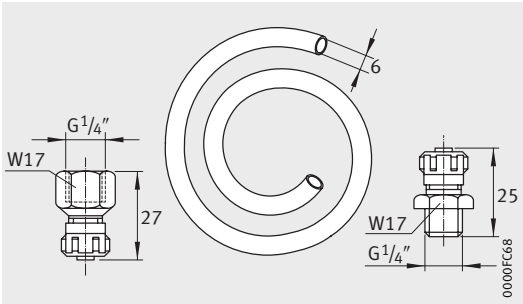
连接油管及接头， 螺母对边宽度 W = 17 mm
