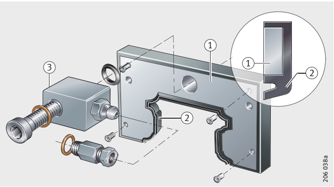
图 10 端部密封件具有单唇密封
