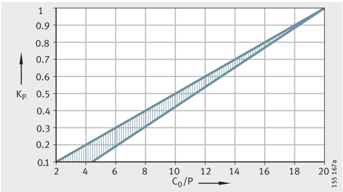
图 3 载荷修正系数
