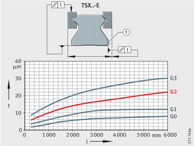
t = 平行度公差 l = 导轨总长度 ① 定位面 图 13 精度等级 和导轨的平行度公差
