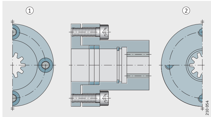
图 1 联轴器
