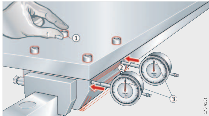
图 20 校直夹紧滑块
