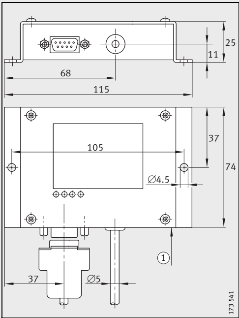
电子评估系统 ASA510 ① 电缆长度 2 m
