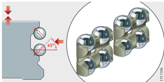
图 1 球兜型保持架
