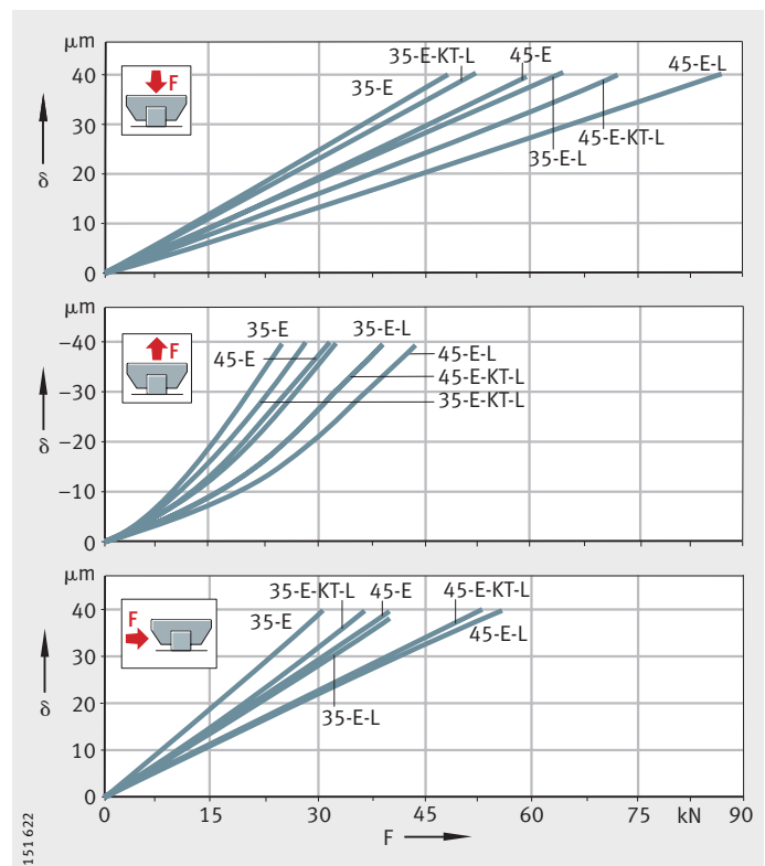
图4 压力、拉力和侧向力作用下的 弹性曲线
