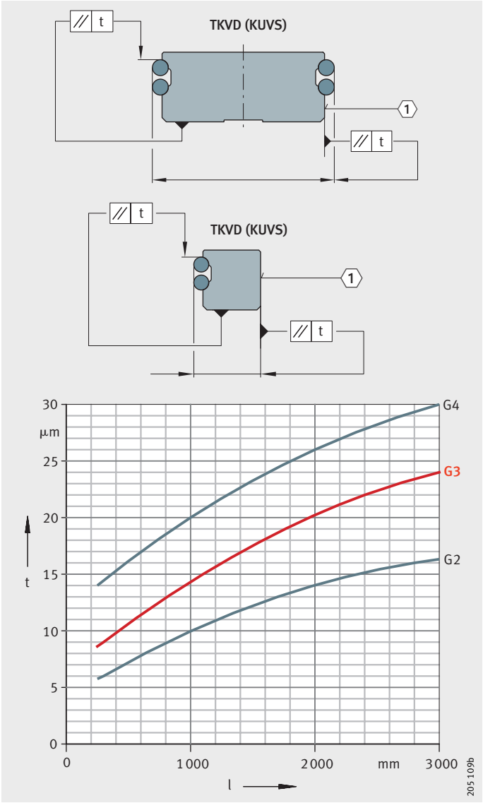
图 8 精度等级 和导轨的平行度公差
