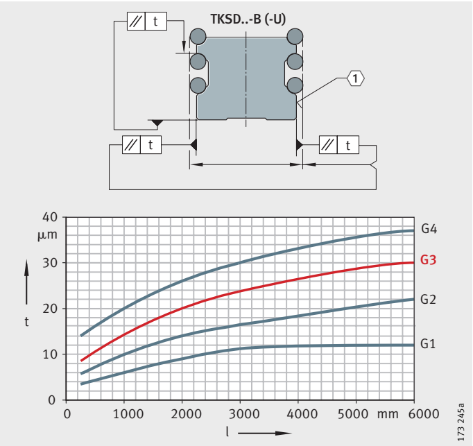
图 11 导轨精度等级和平行度公差
