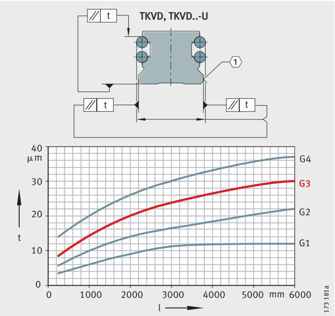
图 26 精度等级 和导轨的平行度公差
