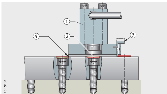
图 10 压入填塞片
