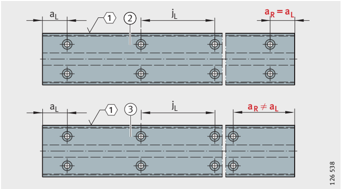
图 3 导轨螺栓孔的形式 两列固定孔
