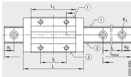
KUVE...-B (-H, -S, -SN) · 视图旋转 90° (1)、(2) 4)
