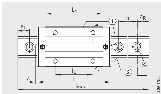
KUSE-H (-HL) · 视图旋转 90° ①、② 4)
