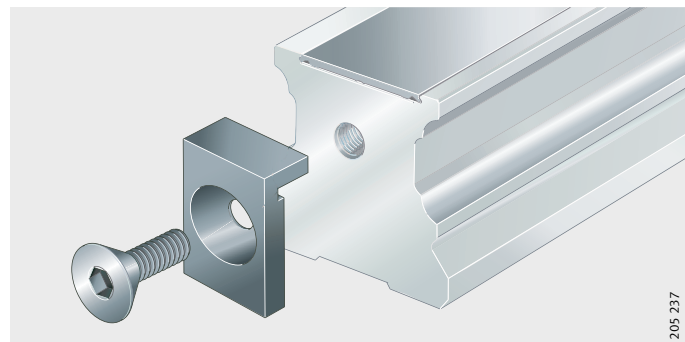
图 4 嵌入式封盖条的固定板
