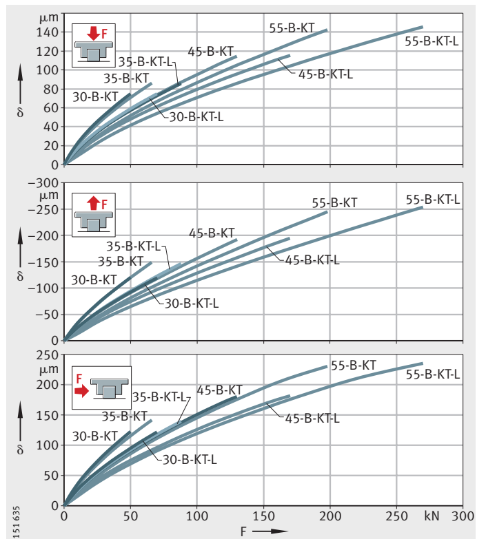
图 19 压力、拉力和侧向力作用下的 弹性曲线
