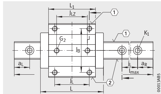
KUBE...B (-L, -N, -NL) · 视图 90° 旋转 ①、② 4)
