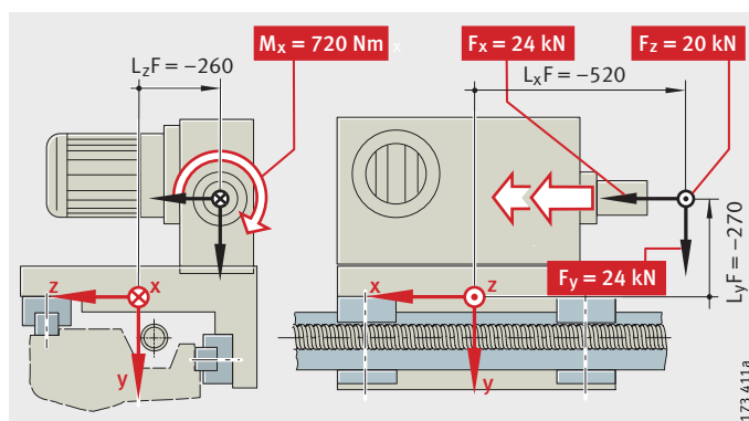
图 8 定义额外的载荷
