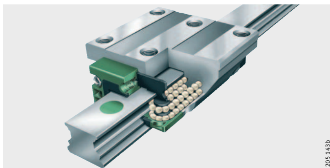
图 4 陶瓷滚动体
