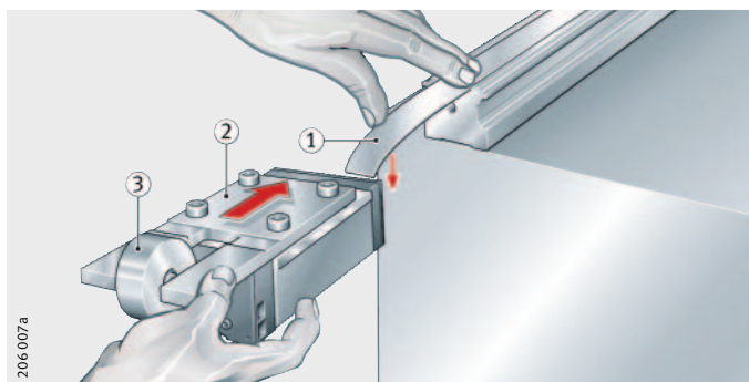
图 18 安装装置安装
