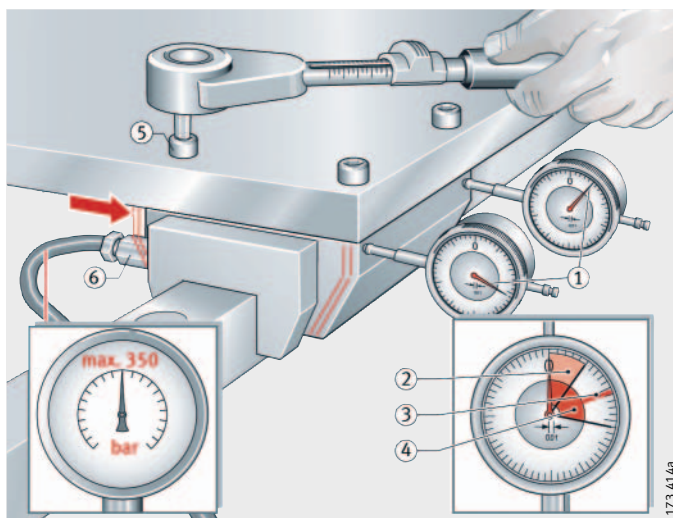
图 21 夹紧滑块安装
