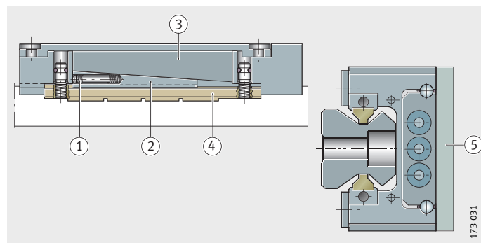
图 11 磨损自动补偿和调整板
