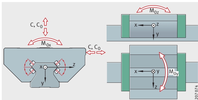
图 1 承载能力和接触角
