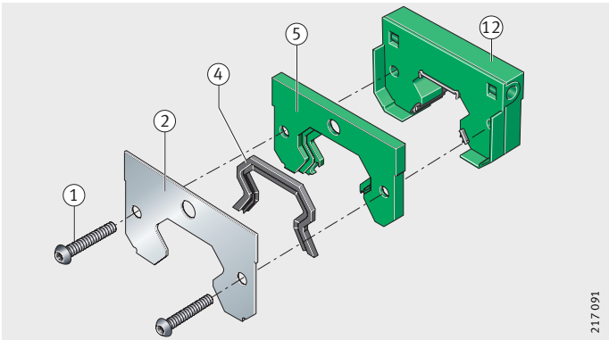
图 8 长效润滑单元
