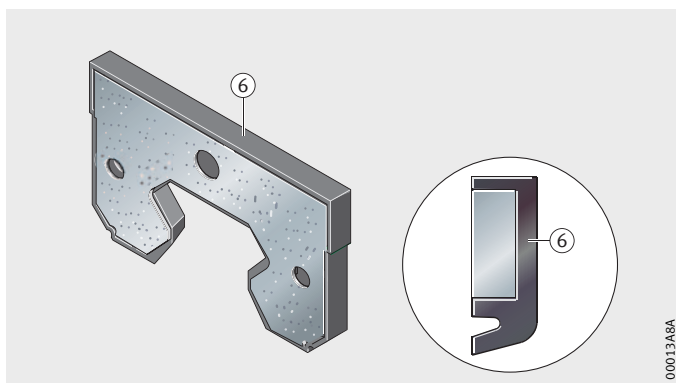
图 5 附加的密封件
