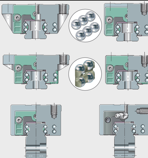
四列直线循环滚珠轴承及导轨组件
