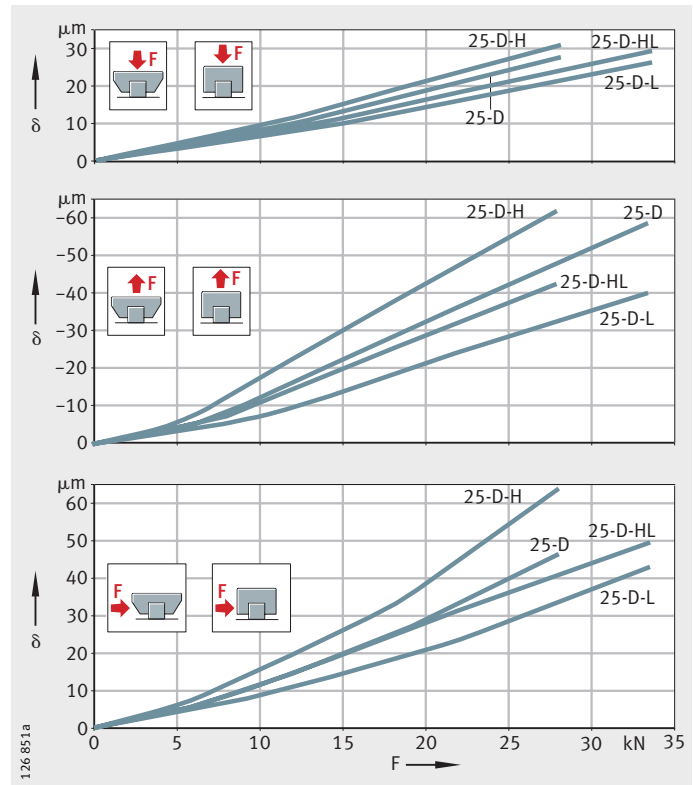
图3 压力、拉力和侧向力作用下的 弹性曲线
