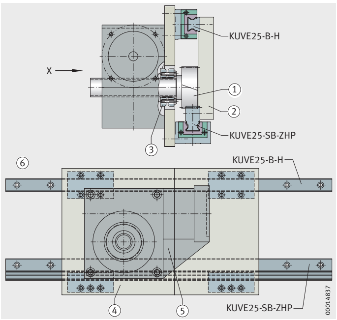
图 13 设计举例
