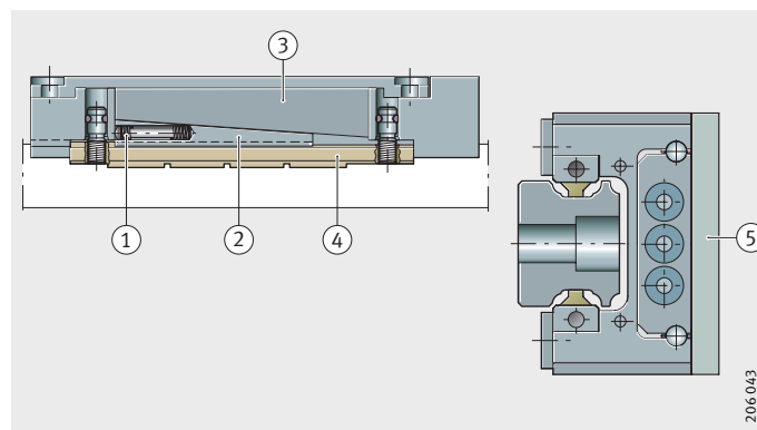
图 7 磨损补偿和调整板
