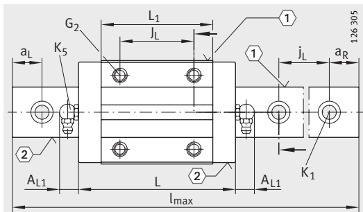
KUE...H 视图旋转 90°
