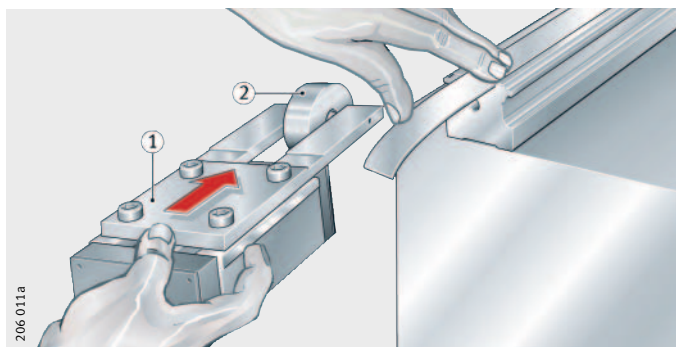
图 19 安装装置安装
