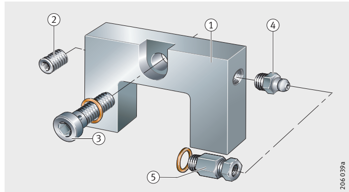
图 12 润滑转接板
