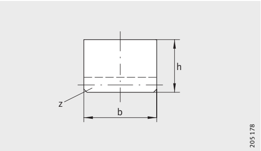
安装配对齿条 MZHP
