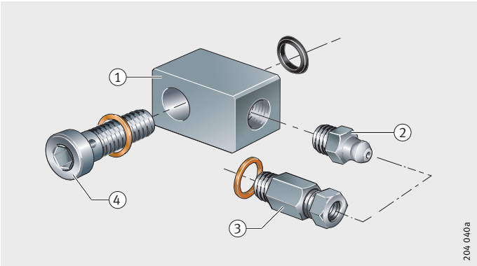
图 4 润滑转接头
