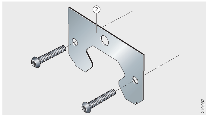
图 1 钢片刮屑片
