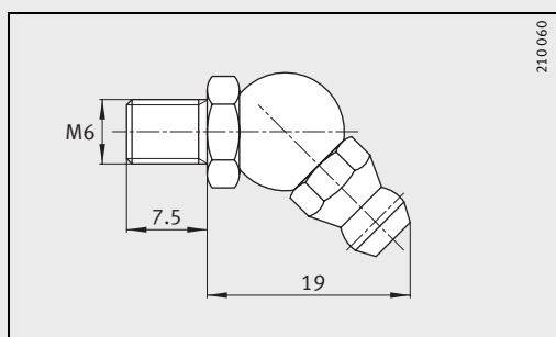
润滑油嘴 3)
