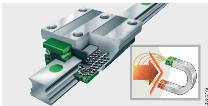
图 2 耐磁钢
