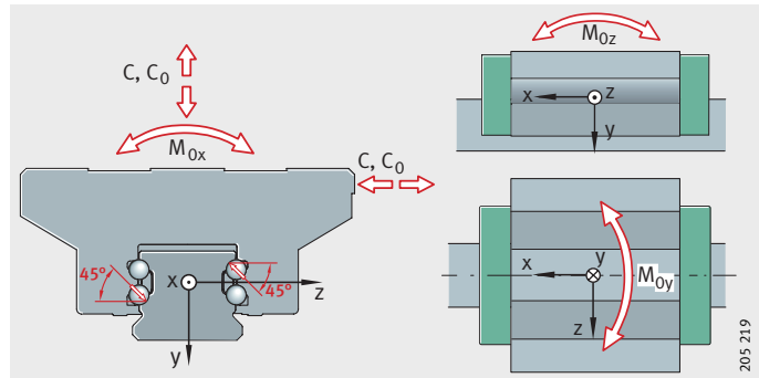
图 2 承载能力和接触角
