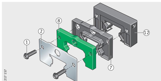
图 6 长效润滑单元
