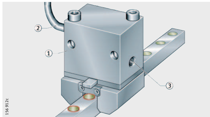
图 9 使用安装装置
