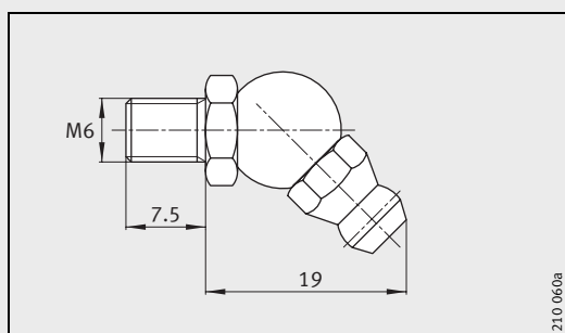
润滑油嘴 2)
