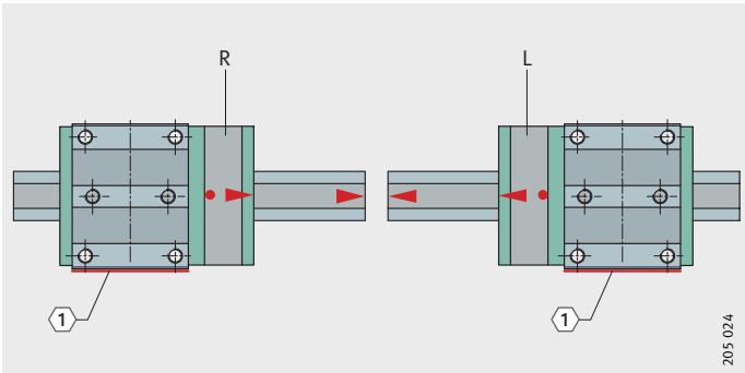
图 6 测量头的位置 (R 或 L) 相对于定位面
