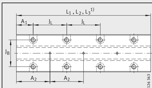
RUDS..-D · 视图旋转 90°
