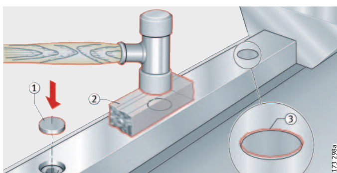
图 6 敲入填塞片
