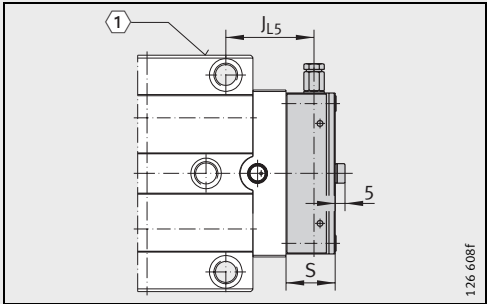
KIT.RWU...-E-511 (-531、-551、-561) 从左边进行再润滑 ① 1)
