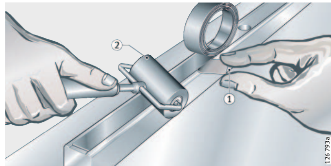
图 15 固定封盖条
