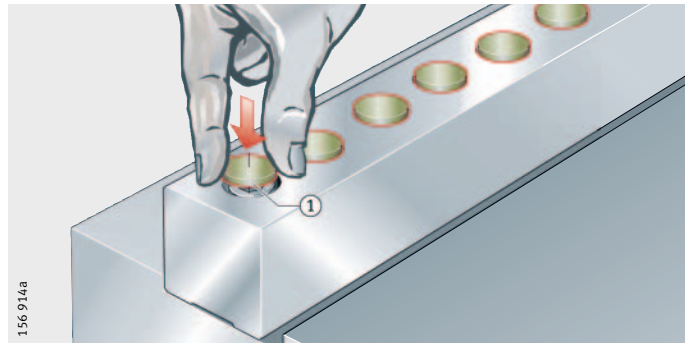
图 8 将填塞片放入沉头孔内
