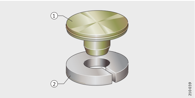
KA..-MSA ① 铜填塞片 ② 塑料固定圈 图 2 带有固定圈的铜填塞片
