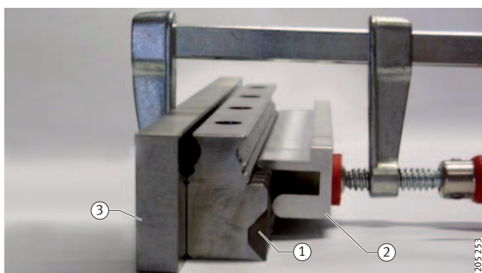
图 7 对齐导轨和齿条
