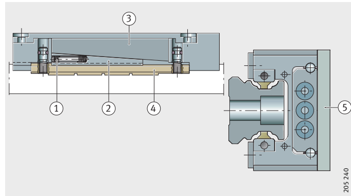
图 9 磨损自动补偿和调整板
