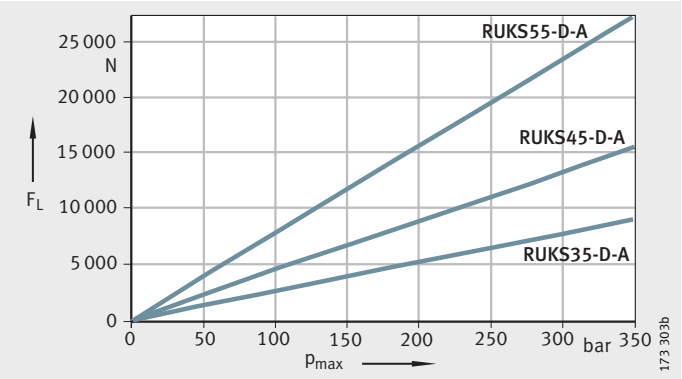
图 8 起步阻力
