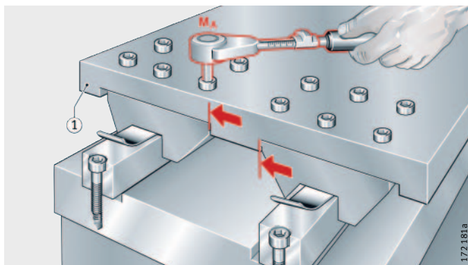
图 26 工作台安装
