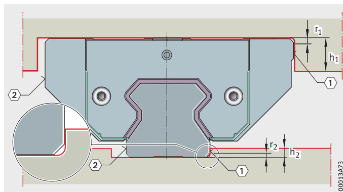
图 2 定位面和标记面
