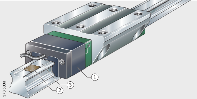
图 1 增量式系统
