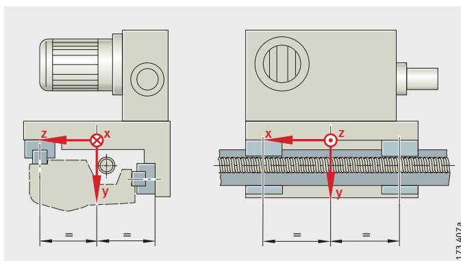
图 4 定义工作台坐标系
