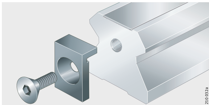
图 5 嵌入式封盖条的固定板
