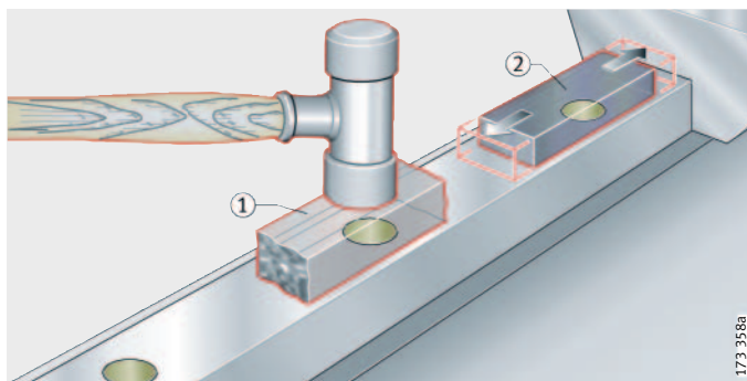
图 7 填塞片的最后安装
