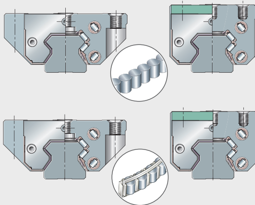
直线循环滚柱轴承及导轨组件
