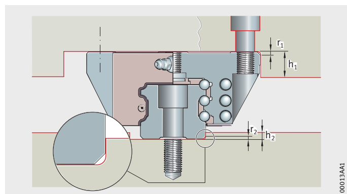
图 10 定位台阶高度和边角半径
