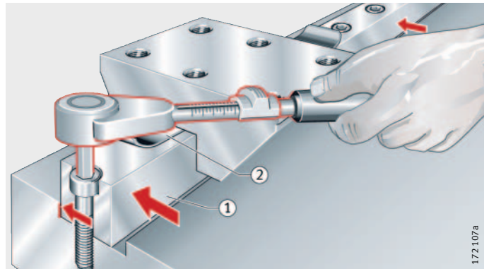
图 24 安装基准端
