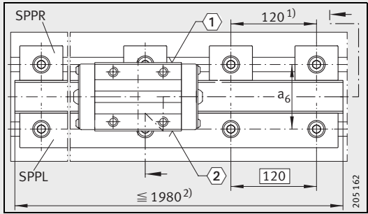
KUVE25-B-K 和 SPPR, SPPL ①、② 3)
