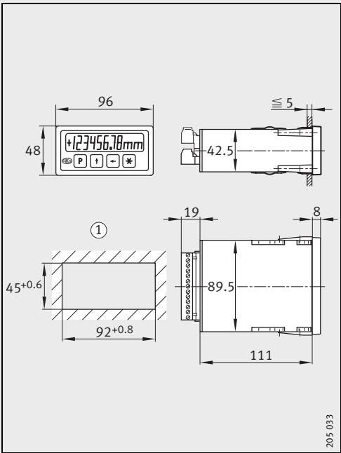
位置显示器 MA10/4（特殊附件） ① 面板外型依据 DIN 43 700
