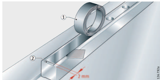
图 14 将封盖条放入槽内
