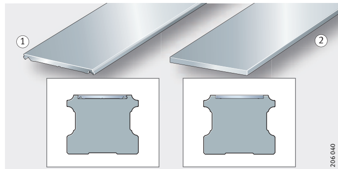
图 2 导轨封盖条
