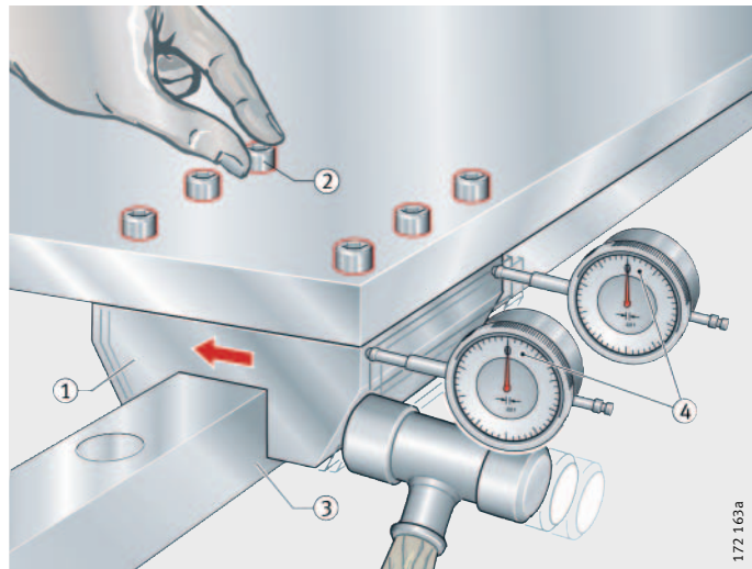
图 22 校正阻尼滑块
