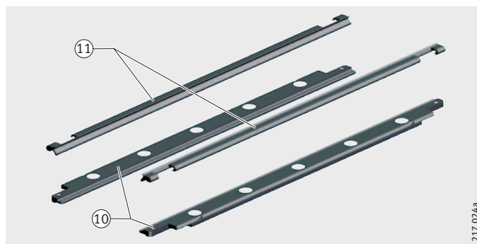
图 5 密封条
