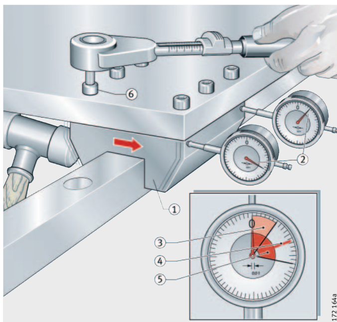
图 23 阻尼滑块安装
