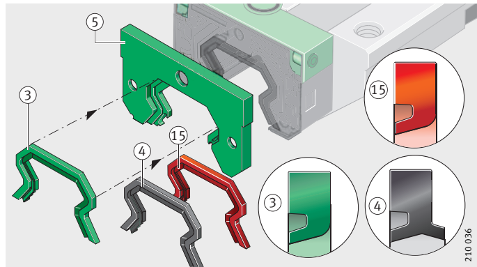
图 3 端部密封件
