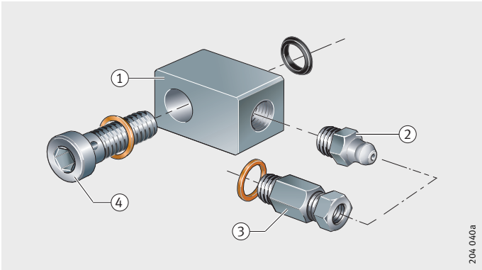
图 11 润滑转接头
