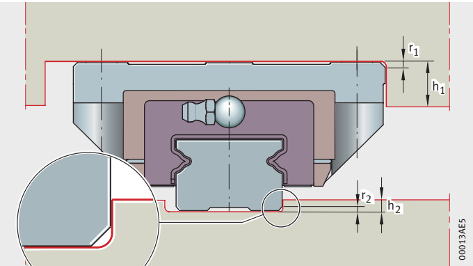
图 6 定位台阶高度和边角半径
