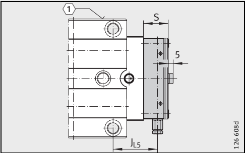
KIT.RWU...-E-510 (-530、-550、-560) 从右边进行再润滑 ① 1)
