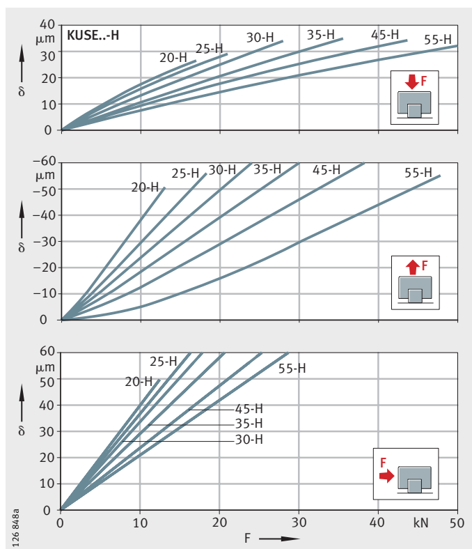
图 5 压、拉及侧向载荷下的弹性曲线
