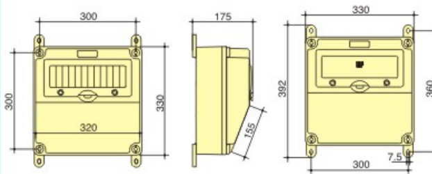
Outline dimension 外形尺寸图
