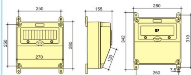
Outline dimension 外形尺寸图
