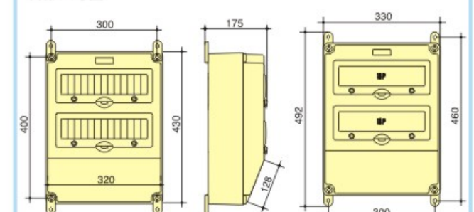
Outline dimension 外形尺寸图
