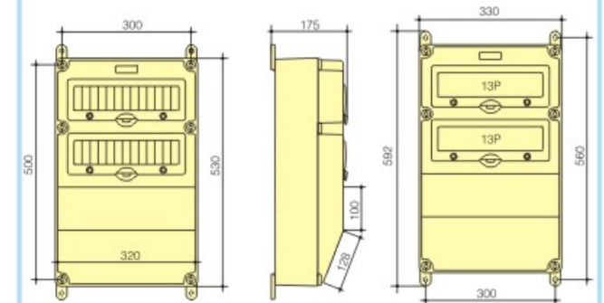
Outline dimension 外形尺寸图
