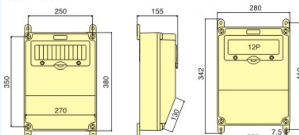
Outline dimension 外形尺寸图
