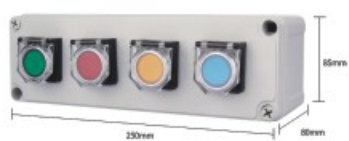
按钮防水盒
