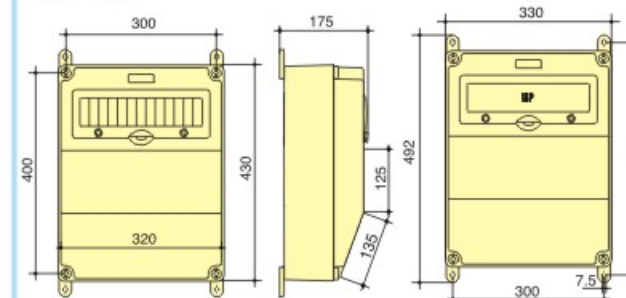
Outline dimension 外形尺寸图
