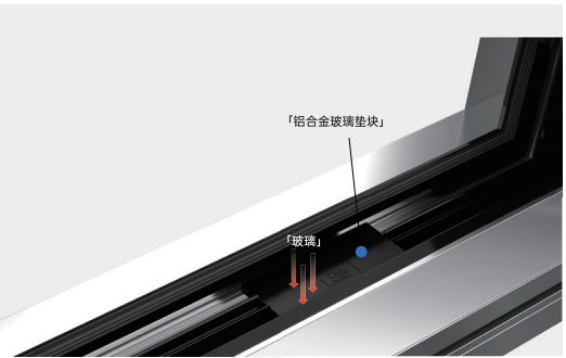
2025年：国内首家使用铝合金玻璃 承重垫块技术
