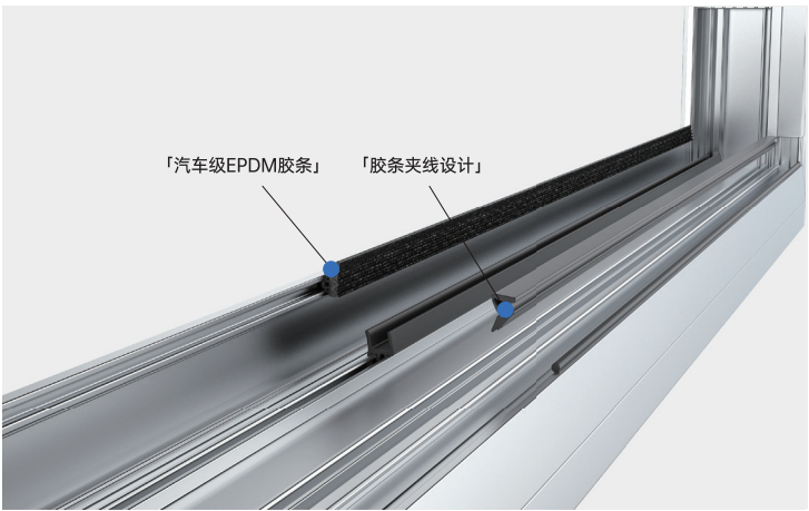
2022年：国内率先使用玻内夹线胶条(不伸缩)技术
